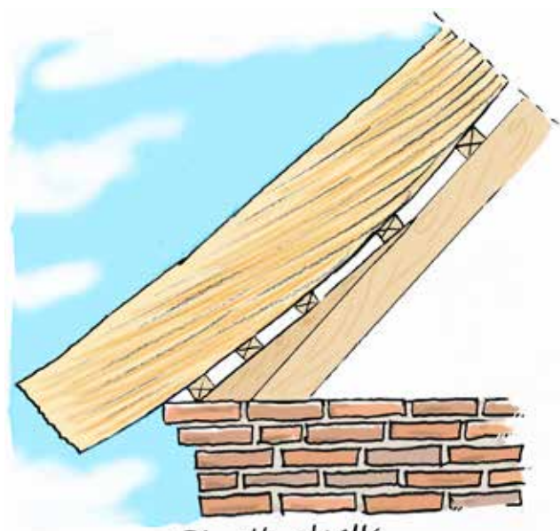
Tegning 31 Opspænd med skjult skalk
