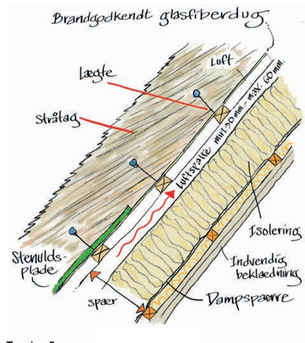
Tegning 5 Brandsikring med glasfiberdug
