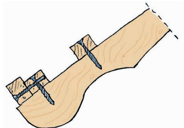
Tegning 29 Forstærket tagskægslægte/bærelægte
