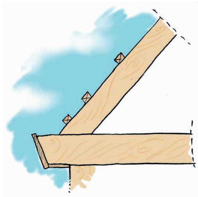
Tegning 34 Stern/sugfjæl
