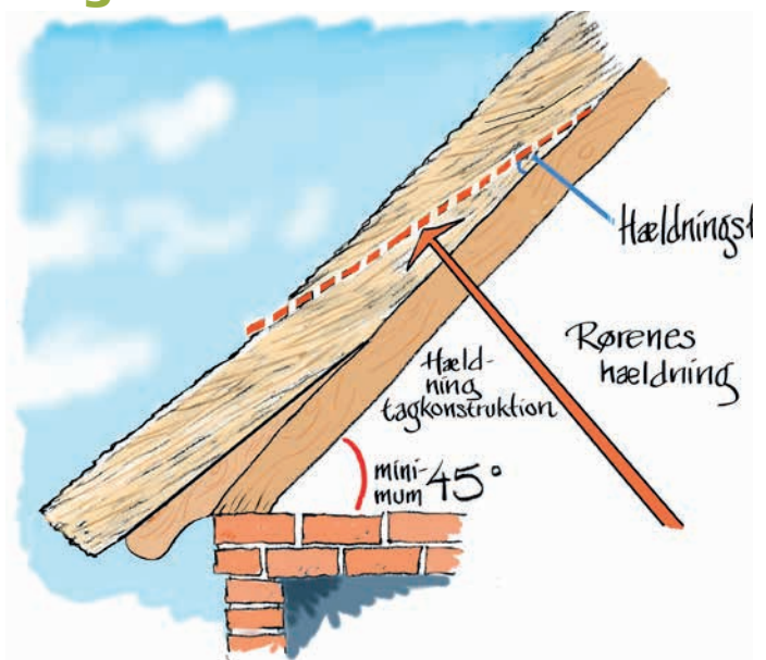
Tegning 6 Hældningstab – Tækkerørene har en lavere hældning end tagkonstruktionen
