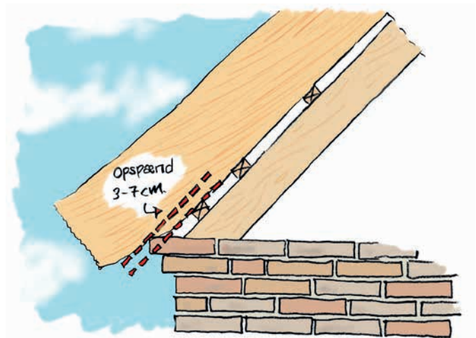
Tegning 35 Muret opspænd ved sternbræt
