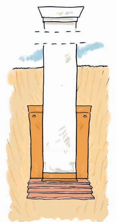
Tegning 51 Inddækning omkring skorsten (front)
