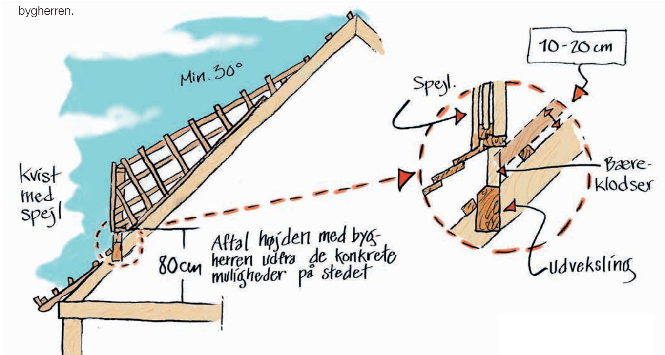
Tegning 39 Snit A i kvist
